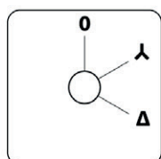
3- PHASE (3 x 0-λ-Δ)
